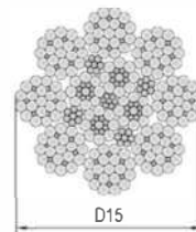
Поперечное сечение талевого каната Wire rope cross section 8x25 Wire Strength 2160 N/mm² 8x25, прочность каната 2160 Н/мм²
