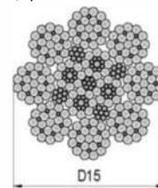
Поперечное сечение талевых канатов Wire rope cross section 8x25, Wire Strength 2160 N/mm² 8x25, прочность каната 2160 Н/мм²
