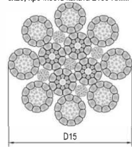
Поперечное сечение талевых канат
