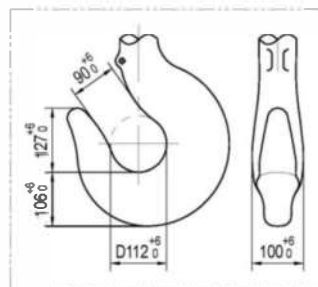
Габариты крюка Hook dimensions DIN 15401-10T
