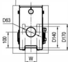
Габариты крюка Hook dimensions DIN15401-5V
