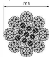
Поперечное сечение талевго каната Wire rope cross section 8x25, Wire Strength 2160 N/mm 2 8x25, прочность каната 2160 Н/мм 2
