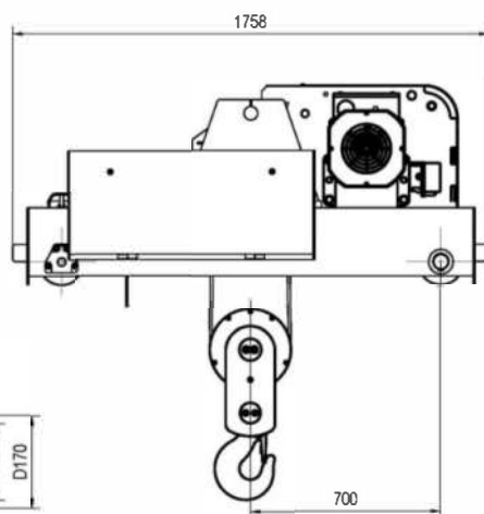
Габариты крюка Hook dimensions DIN15401-5V
