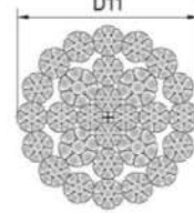
Поперечное сечение талевго каната Wire rope cross section 8x26, Wire Strength 2160 Hkmm (Hsl. ≤18) 8x26, прочность каната 2160 Hkmm (Выс. подъема ≤18)
