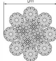
Поперечное сечение талевых канат Wire rope cross section 8x26, Wire Strength 2160 N/mm 2 8x26, прочность каната 2160 Н/мм 2 D11
