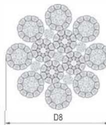
Поперечное сечение талевых канатов Wire rope cross section 8x26, Wire Strength 2160 N/mm 2 (Hol. ≤18) 8x26, прочность каната 2160 N/mm 2 (Выс. подъема ≤ 18)
