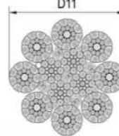
Поперечное сечение талевго каната Wire rope cross section 8x26, Wire Strength 2160 Hkmm (Hsl. ≤18) 8x26, прочность каната 2160 Hkmm (Выс. подъема ≤18)
