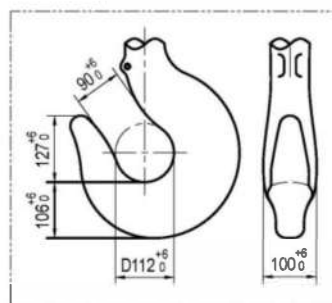
Габариты крюка Hook dimensions DIN15401-10T
