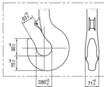
Габариты крюка Hook dimensions DIN15401-5V
